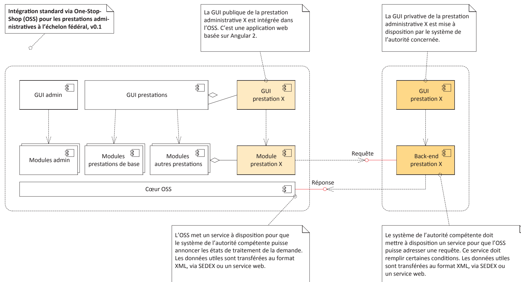
Figure 5: schéma d'intégration
